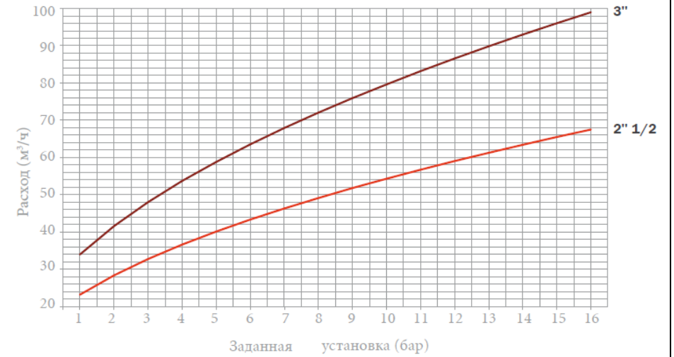
Графики производительности по газу
